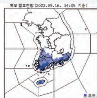
특보현황(9.16. 14시 기준)
