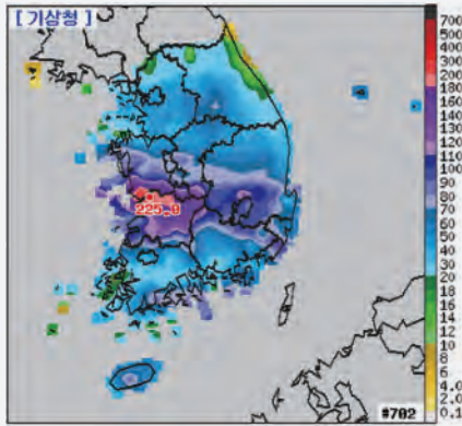
[그림 3-1-7] <5.28.~30. 누적강수량> (출처: 방재기상정보시스템)
