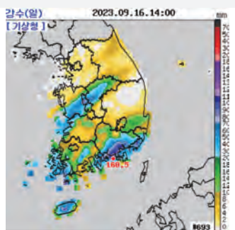
누적강수량(9.16. 14시 기준)
