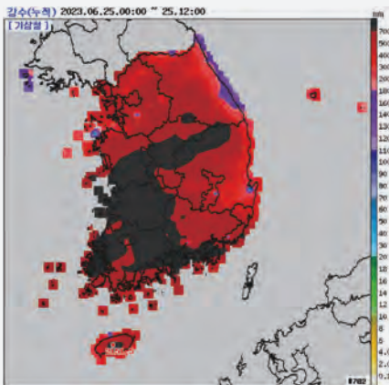
[그림 3-1-9] &lt;'23.6.25~7.25. 누적강수량&gt; (출처: 방재기상정보시스템)
