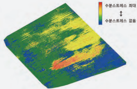
〈이탈리안 라이그라스의 수분스트레스 분포현황〉
