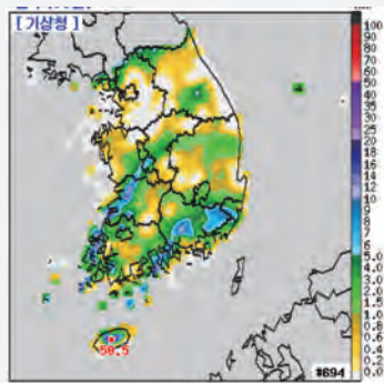
1시간 최대강수량(5.5. 14시)
